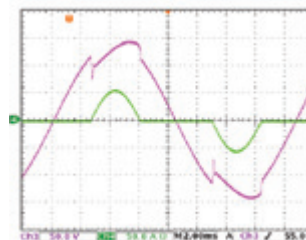
图5: 定电流模式
