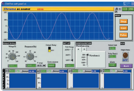
控制主画面
